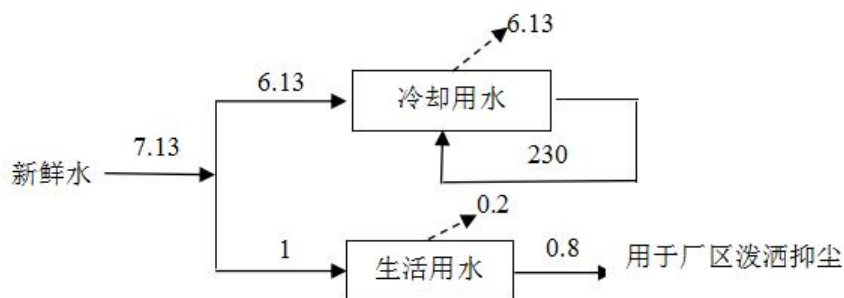
图 2.5-1 项目水平衡图 单位 \text{m}^3/\text{d}
