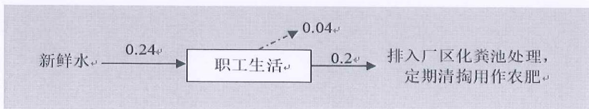
本项目给排水平衡图 单位：m 3 /d
